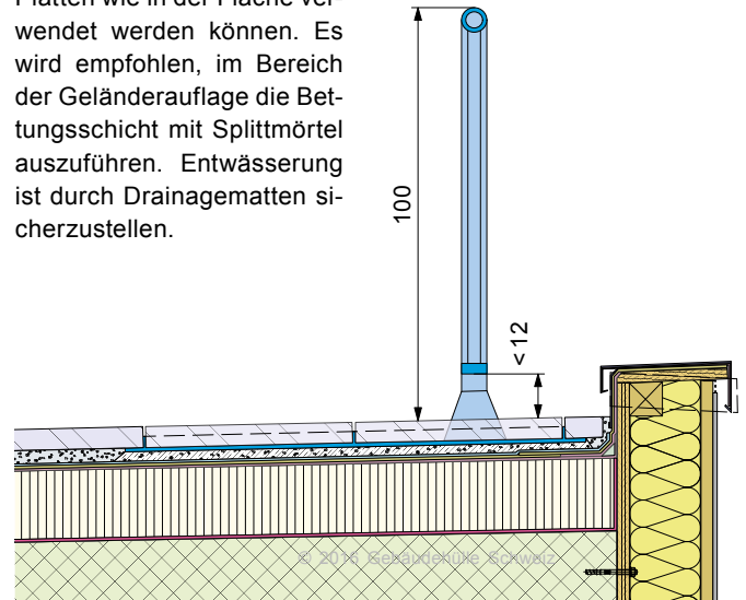
Abb. 19: Systemgeländer mit Auflast der Nuttschicht. Systemanforderungen beachten
