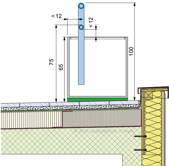
Abb. 18: Pflanztrog auf den Plattenbelag aufgesetzt. Druckfestigkeit der Wärmedämmung (Dauerdruck) ist zu berechnen. Je nach Druck im Bereich des Troges eine Dämmung mit höherer Druckfestigkeit einbauen. Es ist empfehlenswert, solche Pflanztröge linear der Brüstung entlang abzuschotten. Empfehlung bfu: Pflanztröghöhe 75 cm.
